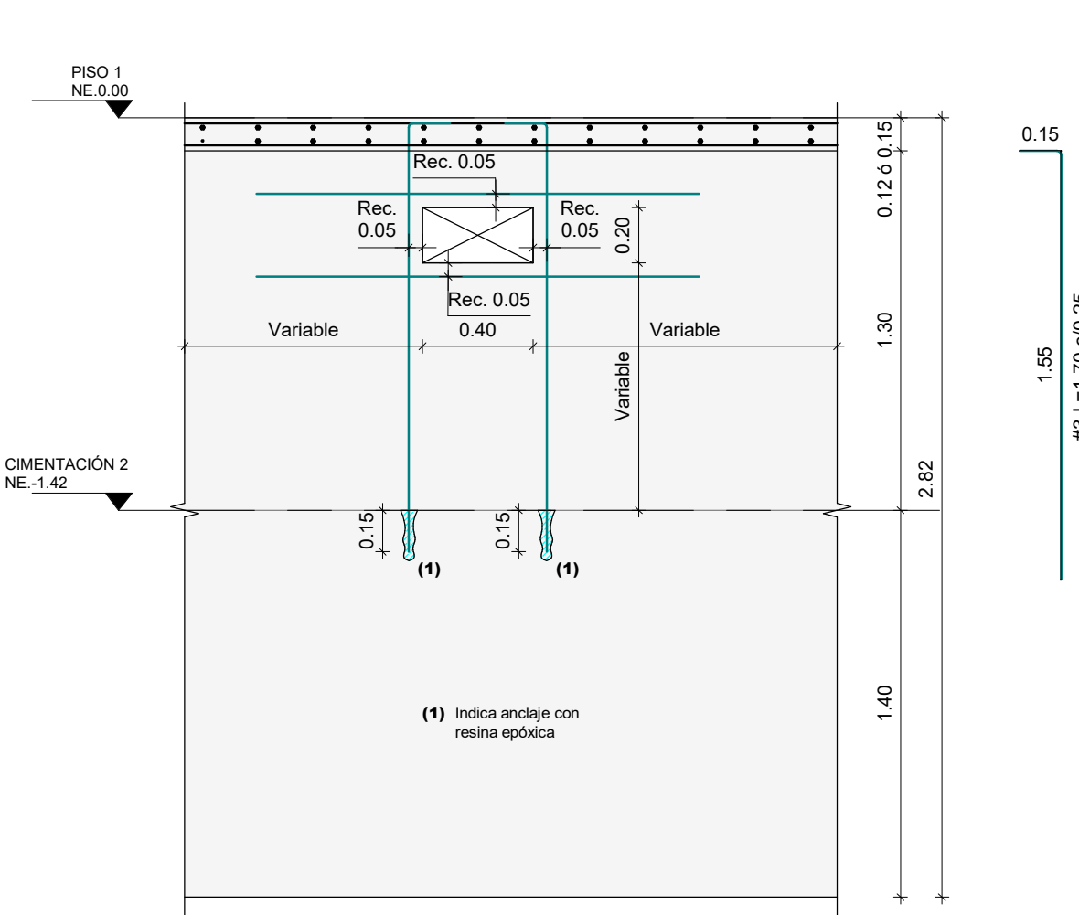
CORTE CIMENTACIÓN Escala 1 : 25
