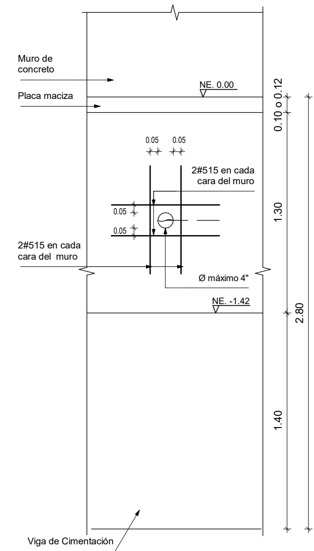
DETALLE PASE MURO Escala 1 : 25
