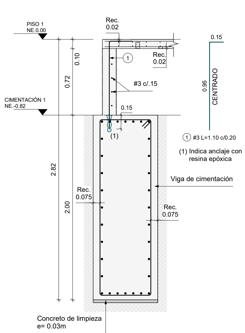
DETALLE MURETE EN CONCRETO TIPO 1 Escala 1 : 25
