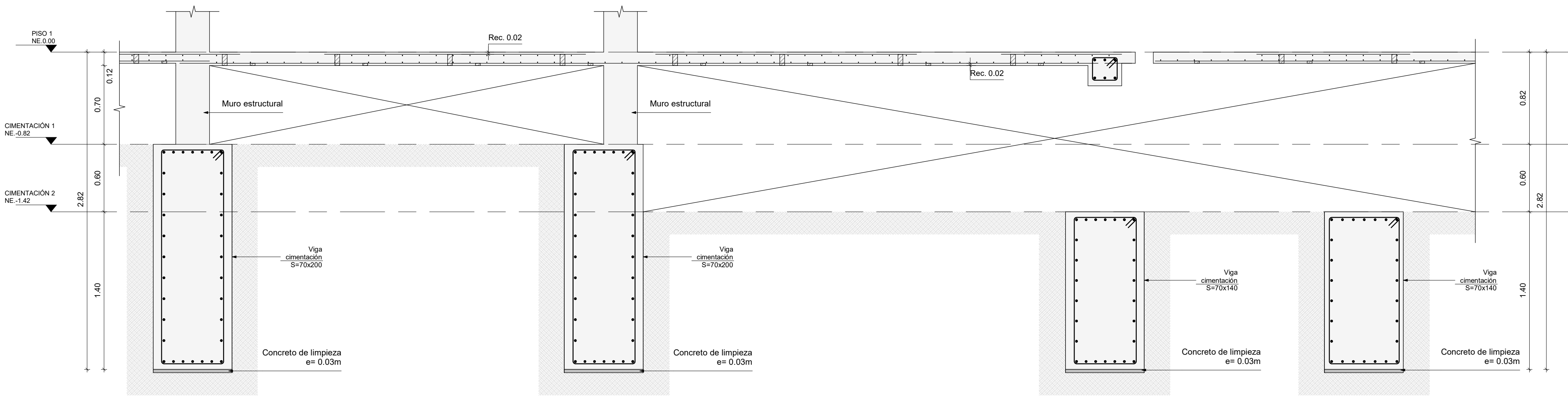
CORTE CIMENTACIÓN Escala 1 : 25
