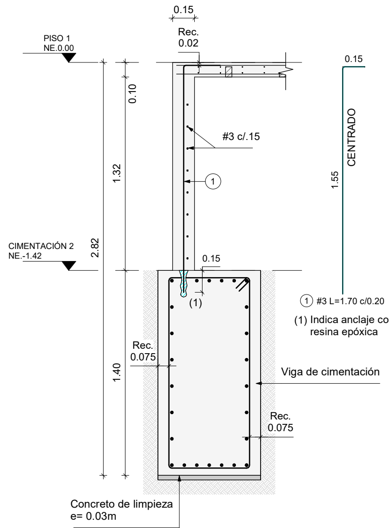
DETALLE MURETE EN CONCRETO TIPO 2 Escala 1 : 25
